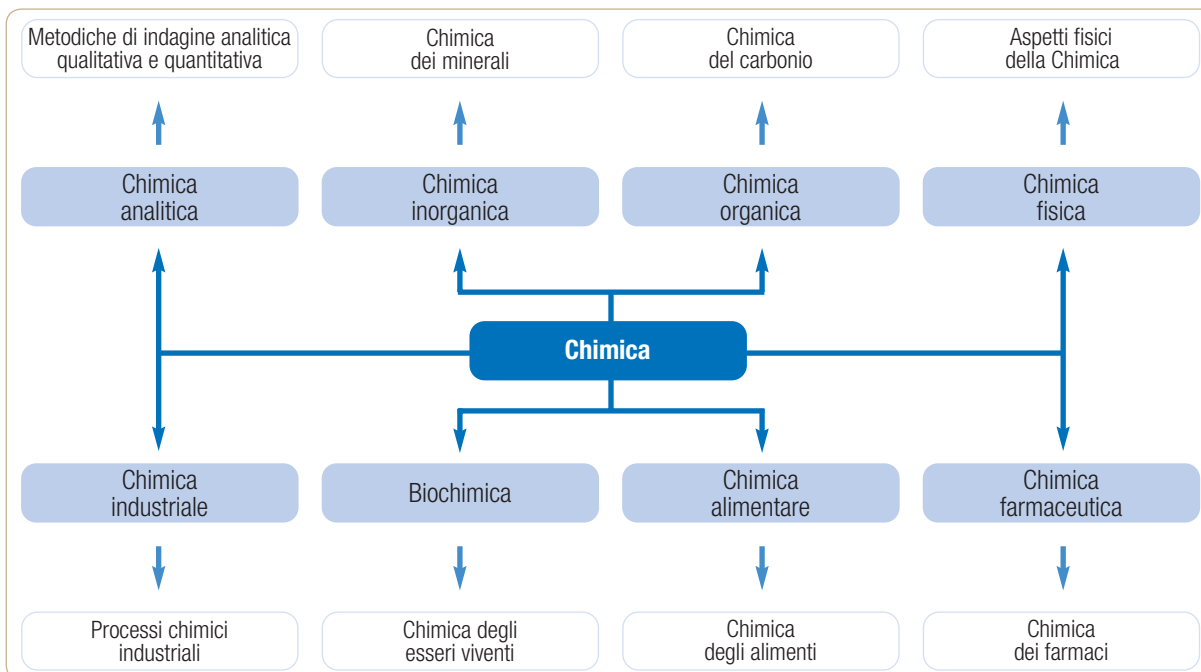
Figura 18 Le branche della Chimica
